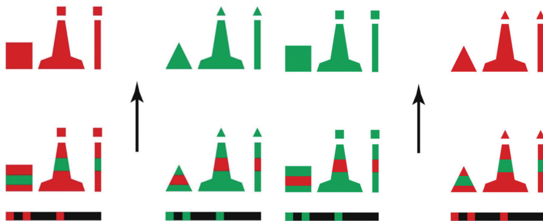
Figura 3.12 - Lateral IALA A e B
